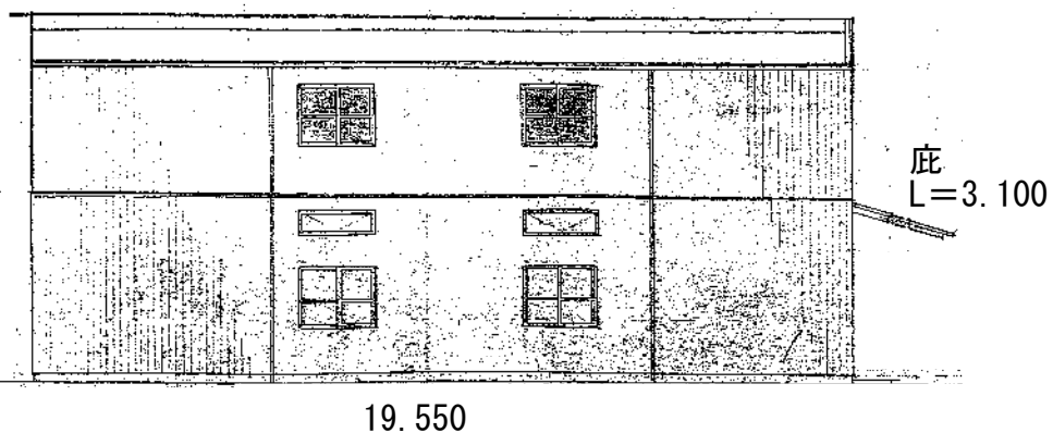
東 立 面 図 S=1/100
