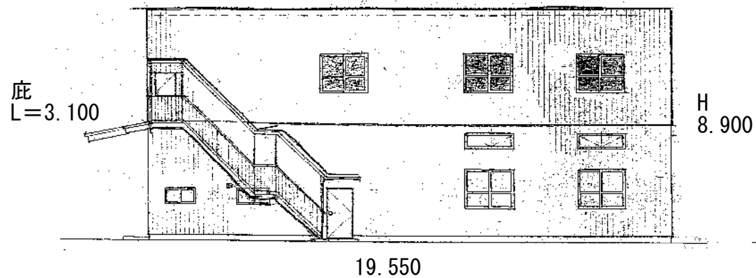
西 立 面 図 S=1/100
