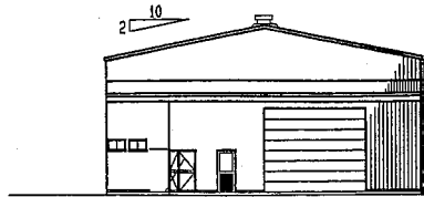
南側立面図 S=1/200
