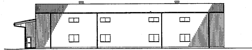
東側立面図 S=1/200
