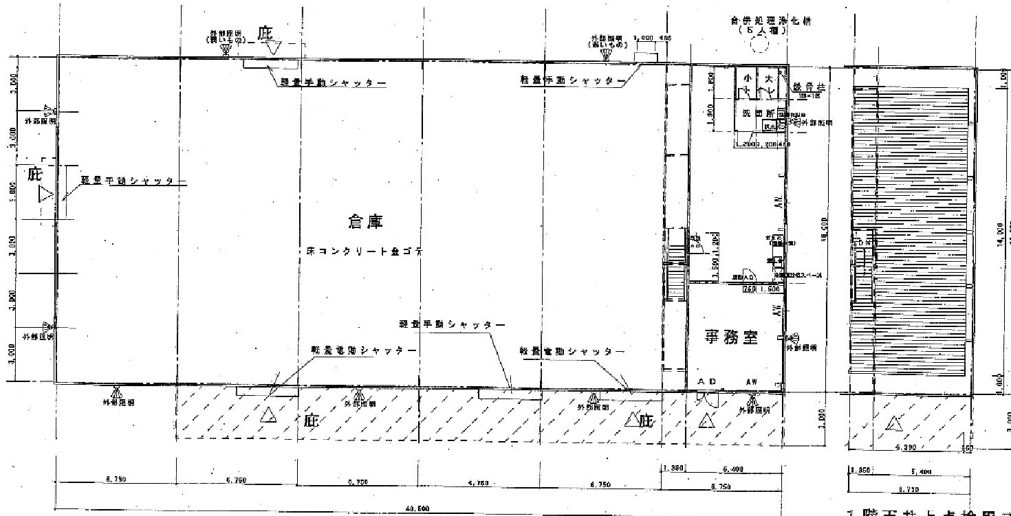
1階平面図
