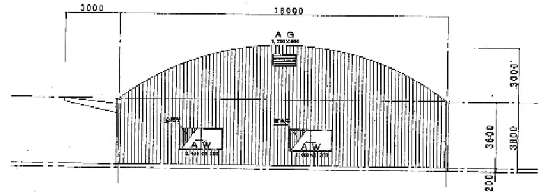
東立面図
