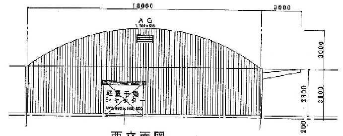
西立面図
